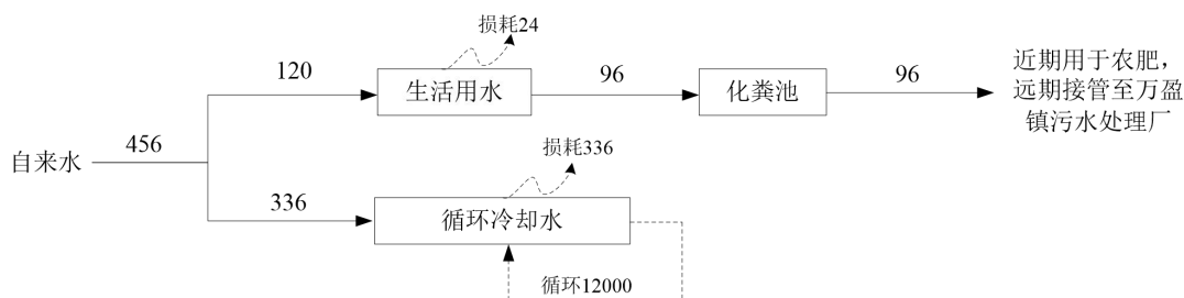
图 2-1 水平衡图（单位：m 3 /a）
